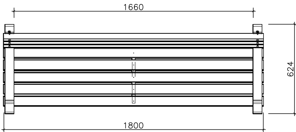
PLANTA TopView
