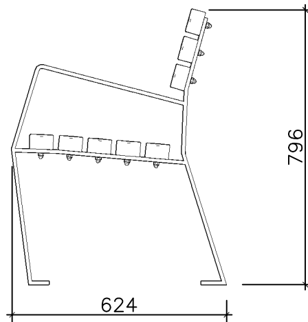
ALÇADO LATERAL Side View
